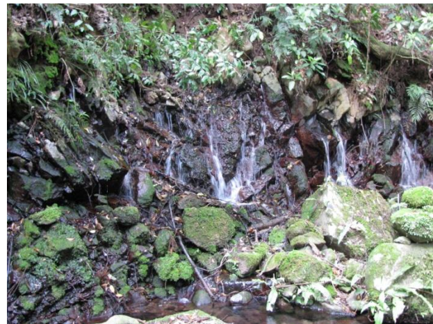
源流は全山地にある
